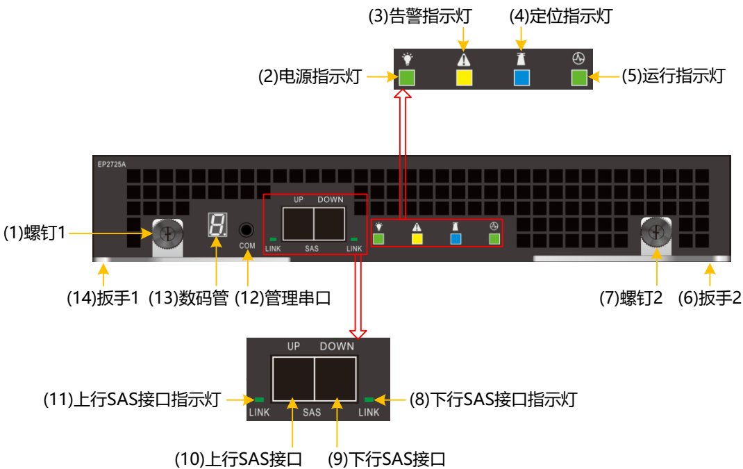
图3-19 DSU2725 的 EP 正视图
