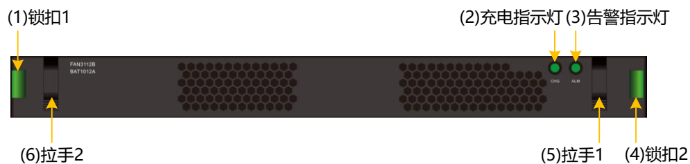
图3-4 SPU 风扇模块+电池模块正视图
