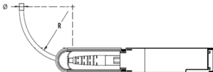
图4-32 AOC 光缆弯曲半径示意图
