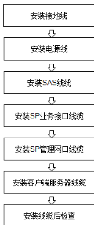
图4-21 线缆安装流程示意图
