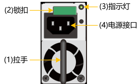
图3-16 DSU2624 电源模块正视图
