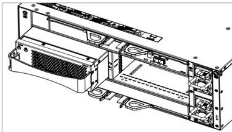
图6-9 安装/拆卸 DSU2624 风扇模块示意图
