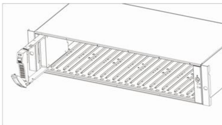
图6-21 安装 2.5 英寸磁盘模块 B 示意图（二）
