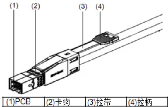
图4-30 SAS 线缆上 Mini SAS HD 连接器示意图
