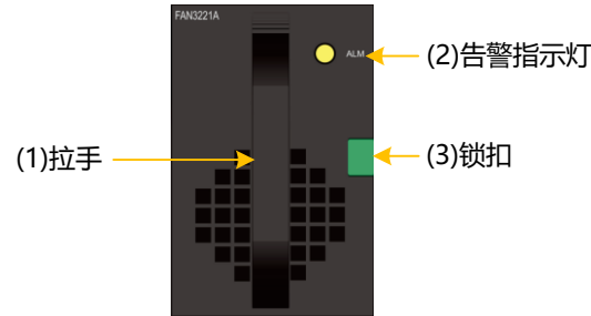
图3-20 DSU2725 后端风扇模块正视图
