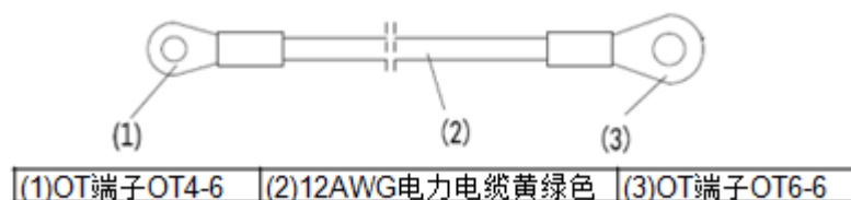
图4-22 接地线示意图
