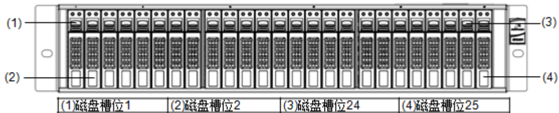
图6-15 DSU2625 磁盘槽位编号示意图
