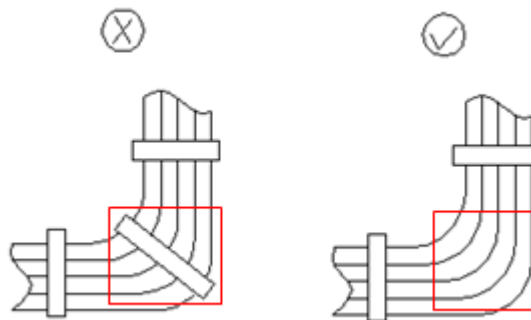
图4-20 线缆捆扎示意图（三）
