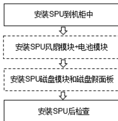
图4-12 SPU 安装流程示意图
