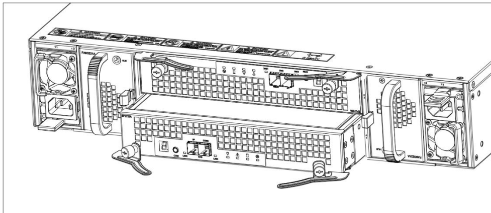
图6-7 安装/拆卸 DSU2725 EP 示意图
