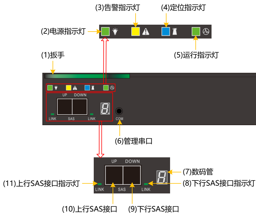
图3-9 DSU2625 的 EP 正视图
