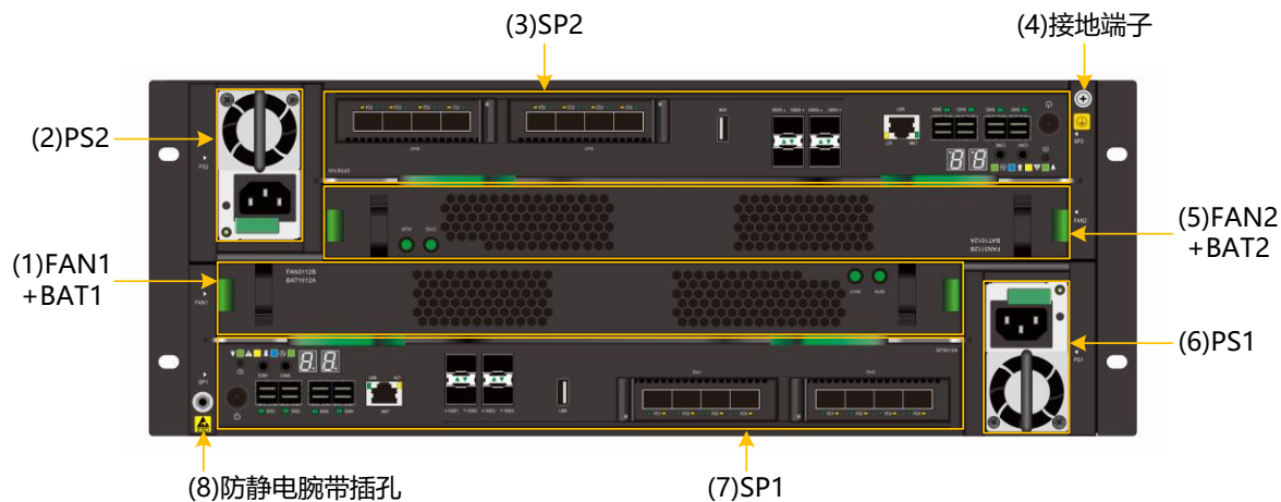
图3-2 SPU 后正视图
