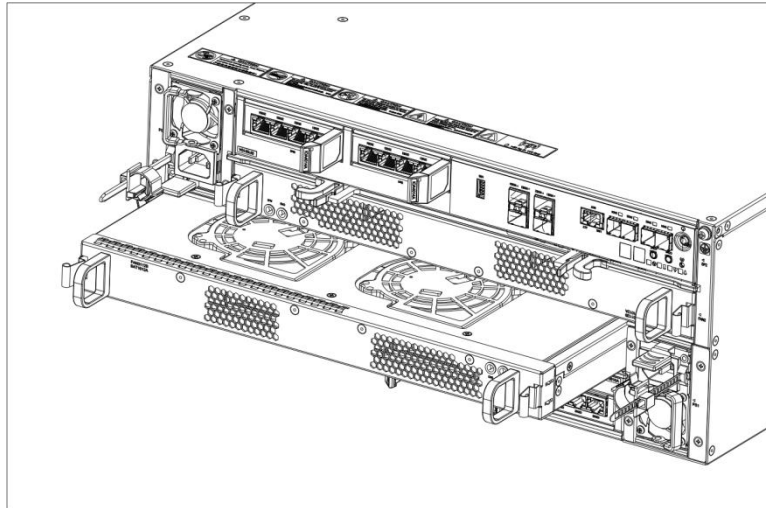
图6-2 安装/拆卸 SPU 风扇模块+电池模块示意图
