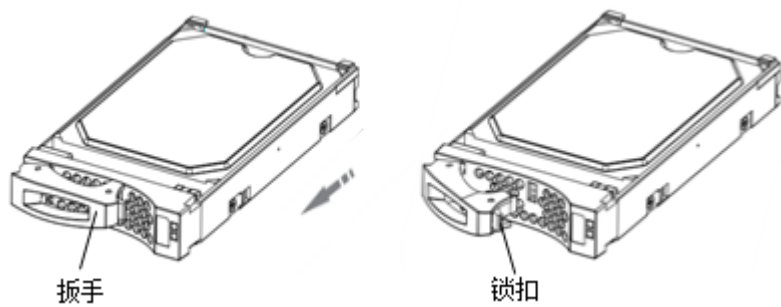
图6-24 安装 3.5 英寸磁盘模块示意图（一）
