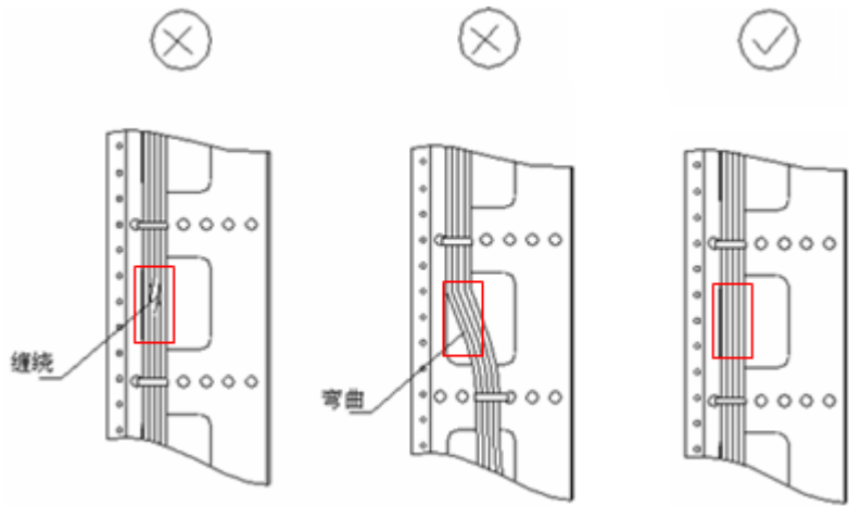
图4-18 线缆捆扎示意图（一）
