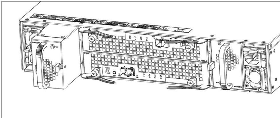
图6-10 安装/拆卸 DSU2725 后端风扇模块示意图
