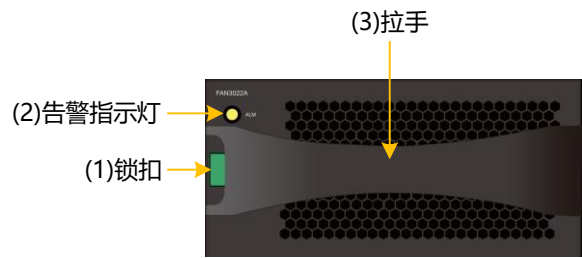
图3-15 DSU2624 风扇模块正视图
