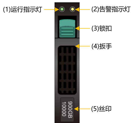
图3-26 2.5 英寸磁盘模块前面板
