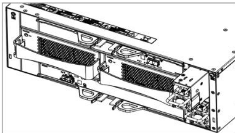
图图 6-13 安装/拆卸 DSU2624 电源模块示意图
