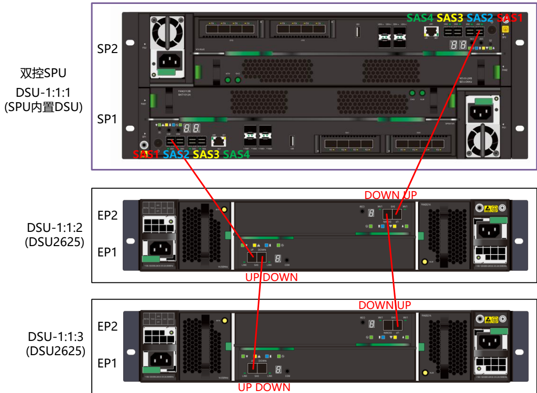
图4-33 SAS 线缆安装示意图
