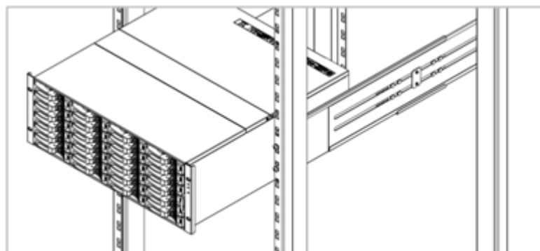
图4-16 安装 DSU 示意图
