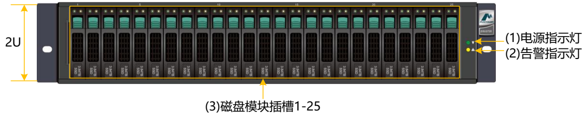
图3-17 DSU2725 前正视图
