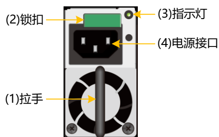
图3-23 DSU2725 电源模块正视图
