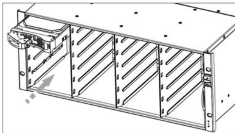
图6-25 安装 3.5 英寸磁盘模块示意图（二）
