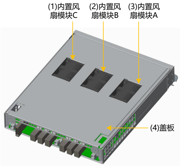
图3-21 DSU2725 内置风扇模块安装位置示意图
