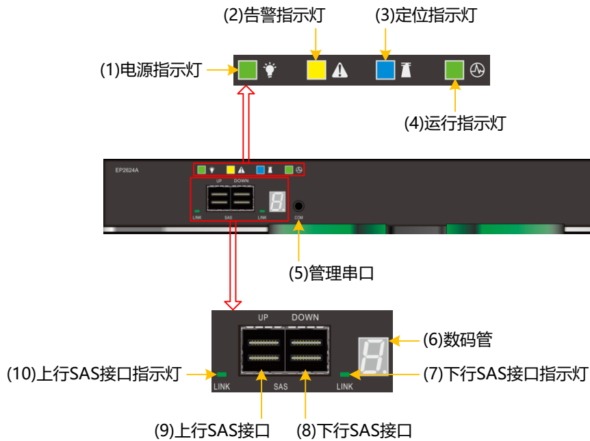
图3-14 DSU2624 的 EP 正视图
