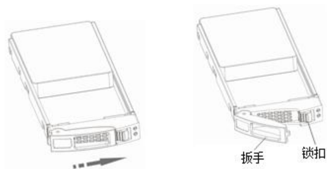
图6-20 安装 2.5 英寸磁盘模块 B 示意图（一）
