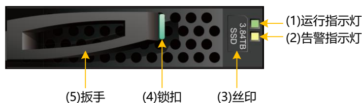
图3-27 3.5 英寸磁盘模块前面板
