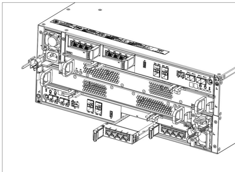
图6-4 安装/拆卸 IO 插卡示意图
