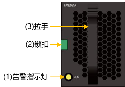
图3-10 DSU2625 风扇模块正视图
