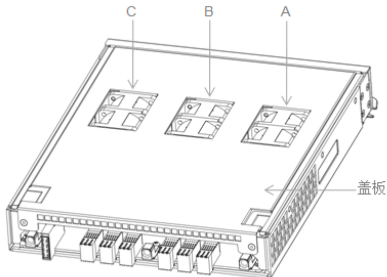
图6-11 DSU2725 内置风扇模块安装位置示意图
