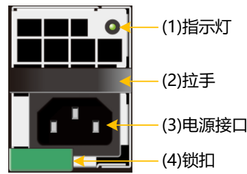
图3-11 DSU2625 电源模块正视图
