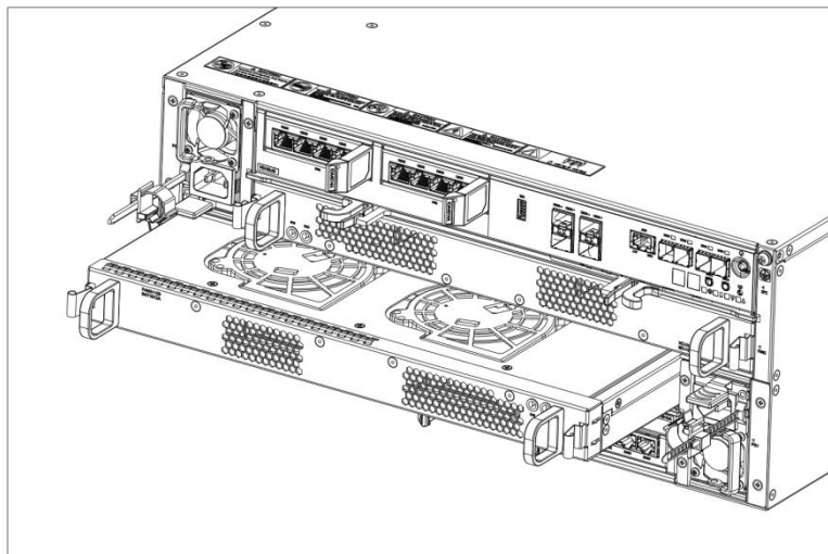
图4-14 安装 SPU 风扇模块+电池模块示意图
