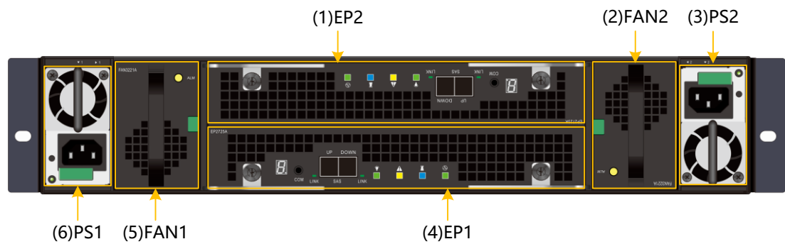
图3-18 DSU2725 后正视图
