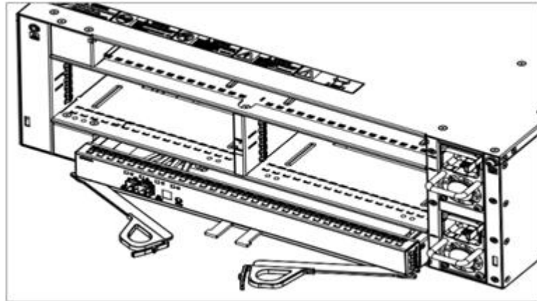
图6-6 安装/拆卸 DSU2624 EP 示意图
