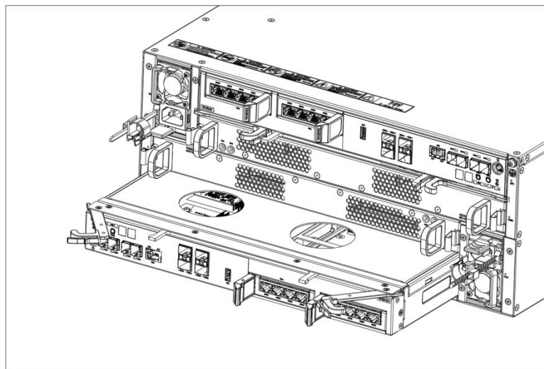
图6-1 安装/拆卸 SP 示意图
