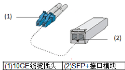
图4-37 10GE 线缆和接口示意图
