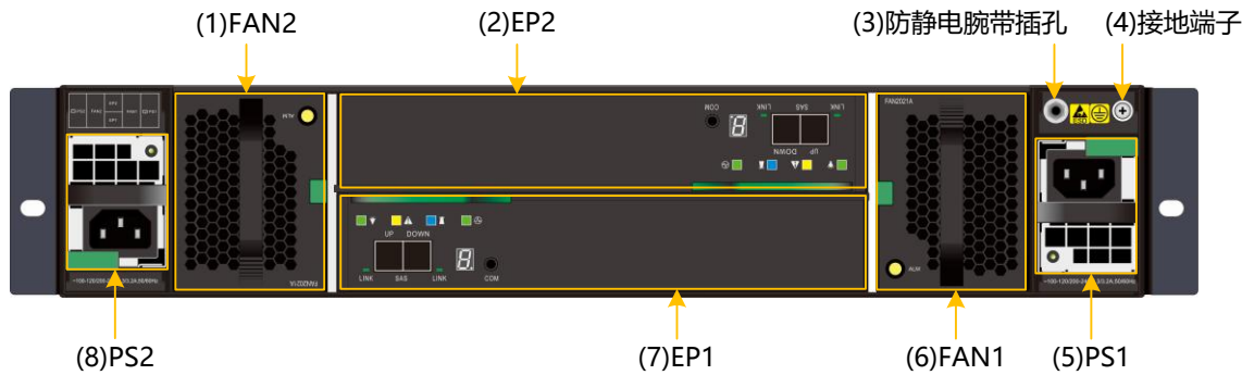
图3-8 DSU2625 后正视图
