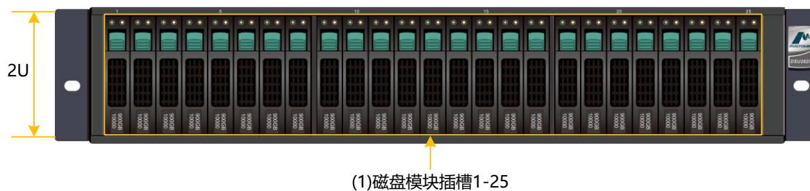
图3-7 DSU2625 前正视图
