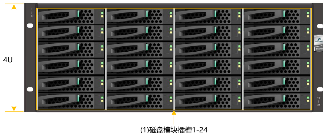
图3-1 SPU 前正视图
