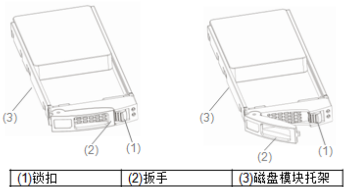
图6-18 2.5 英寸磁盘模块 B 示意图
