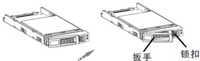
图6-16 安装 2.5 英寸磁盘模块 A 示意图（一）
