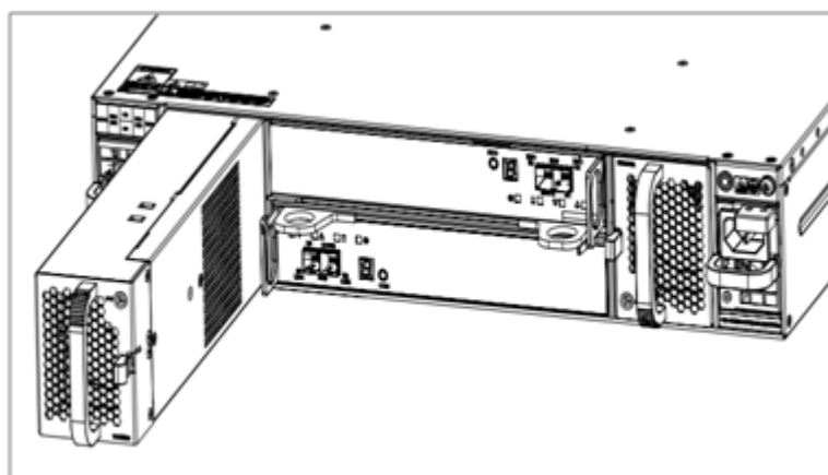
图6-8 安装/拆卸 DSU2625 风扇模块示意图
