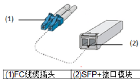
图4-35 FC 线缆和接口示意图
