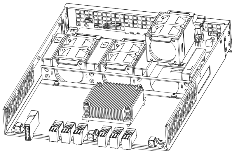
图6-12 安装/拆卸 DSU2725 内置风扇模块示意图
